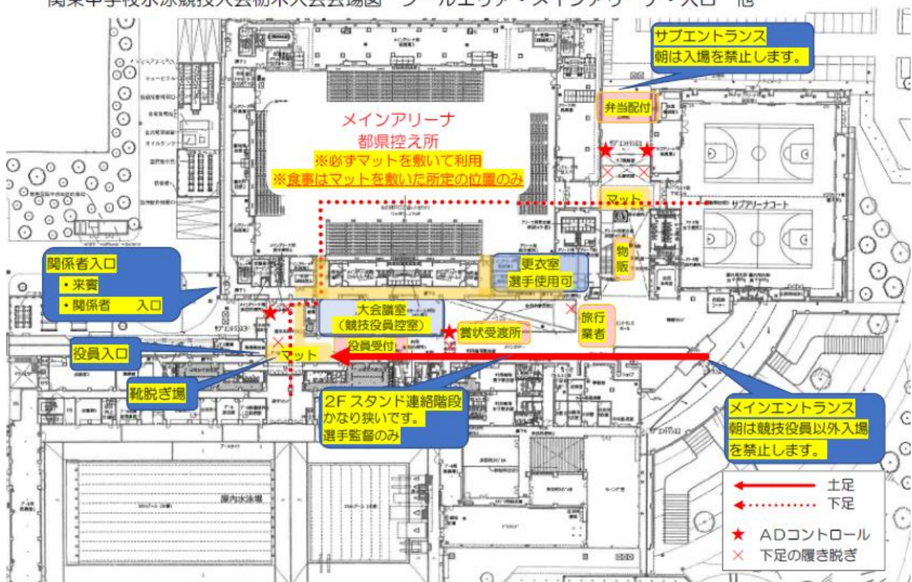
関東中学校水泳競技大会栃木大会会場図 プールエリア・メインアリーナ・入口 他
